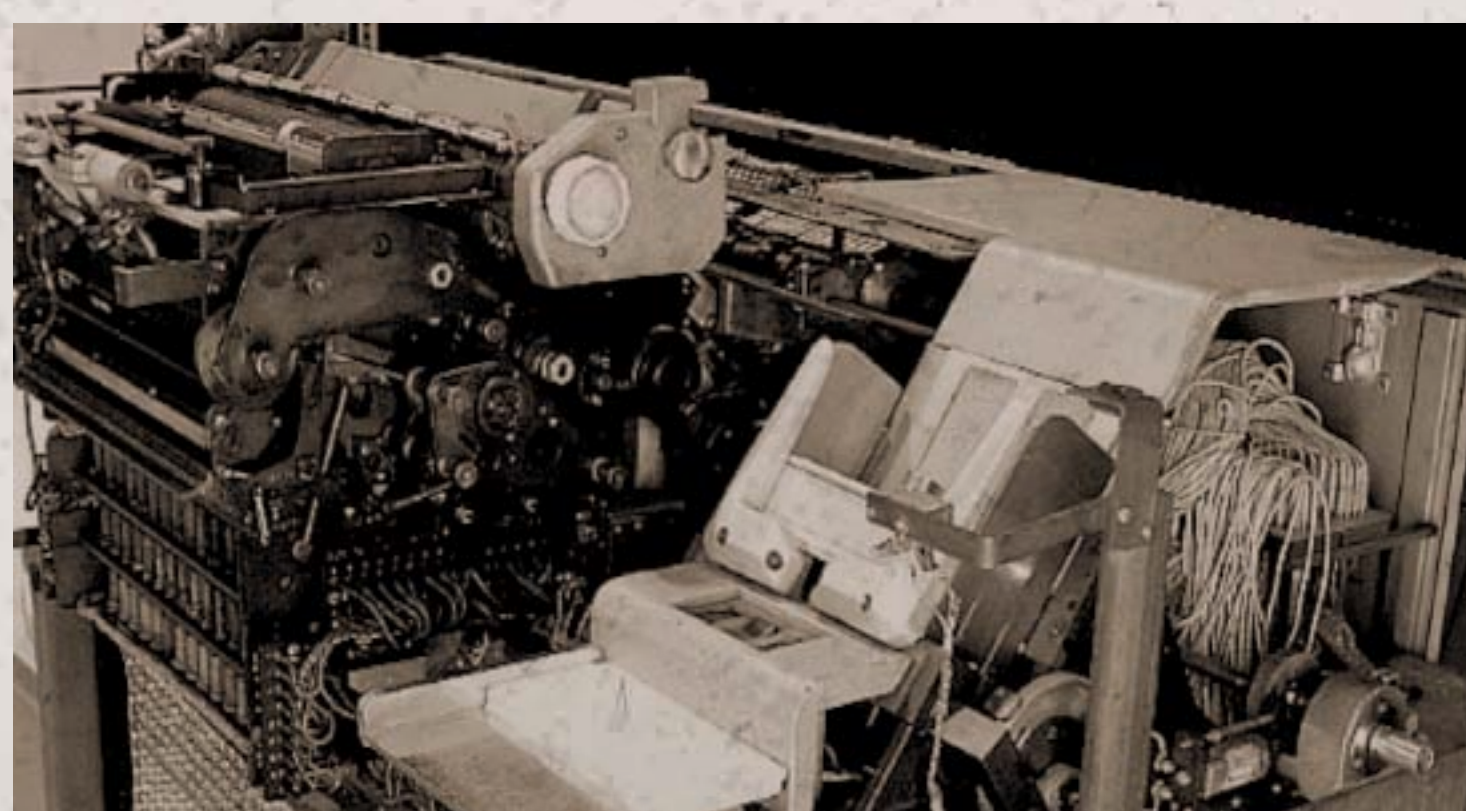
Wnętrze tabulatora
