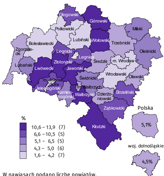
Mapa 1. Stopa bezrobocia rejestrowanego według powiatów w listopadzie 2019 r. (stan w końcu miesiąca)
