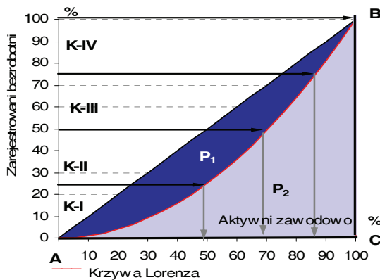
Krzywa koncentracji (krzywa Lorenza)
